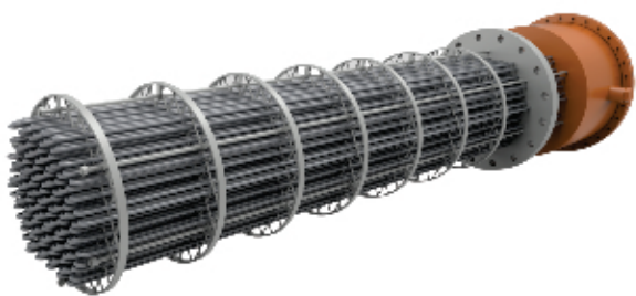
Rod Type Baffles
